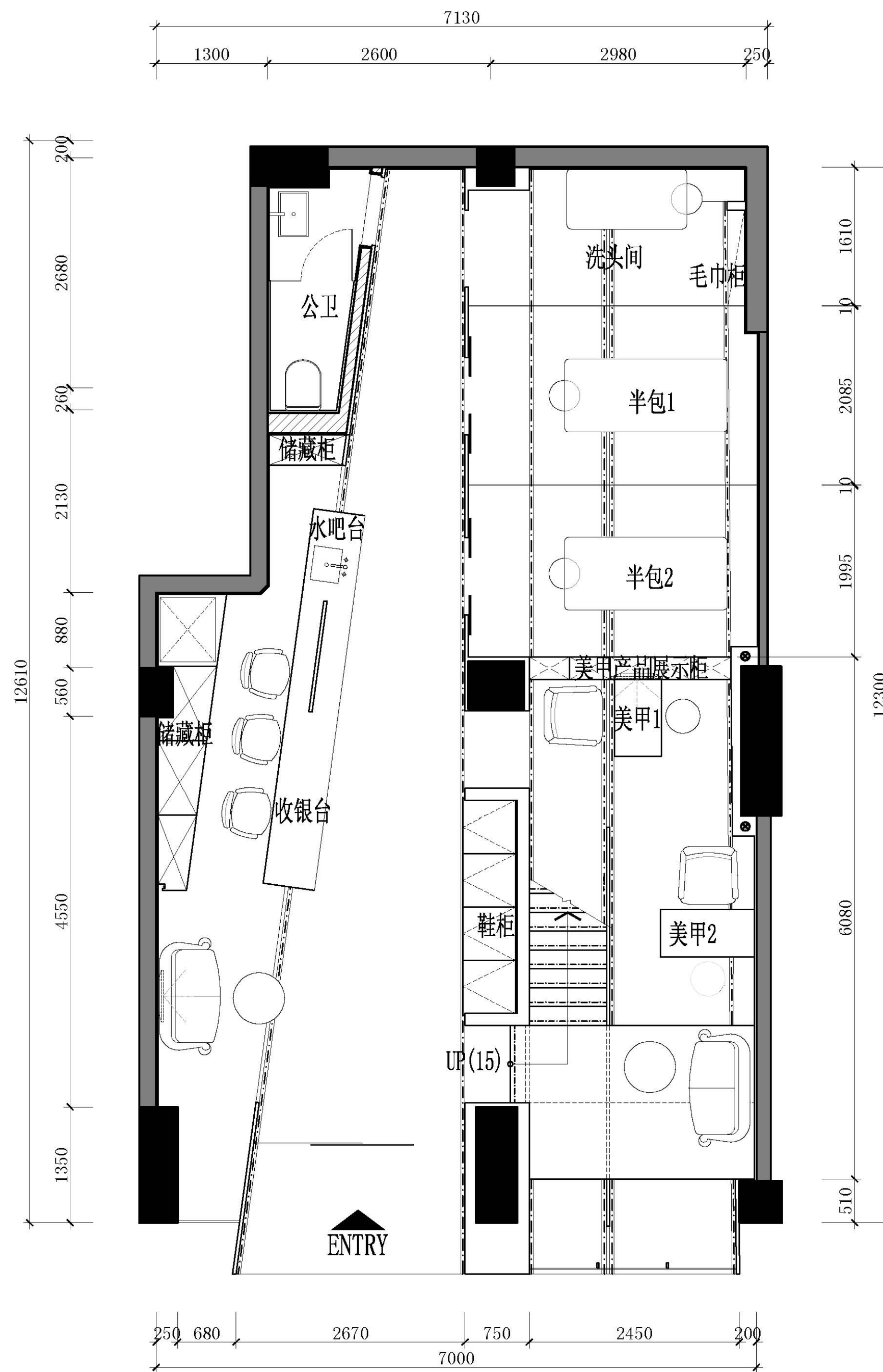
一层平面布置图
